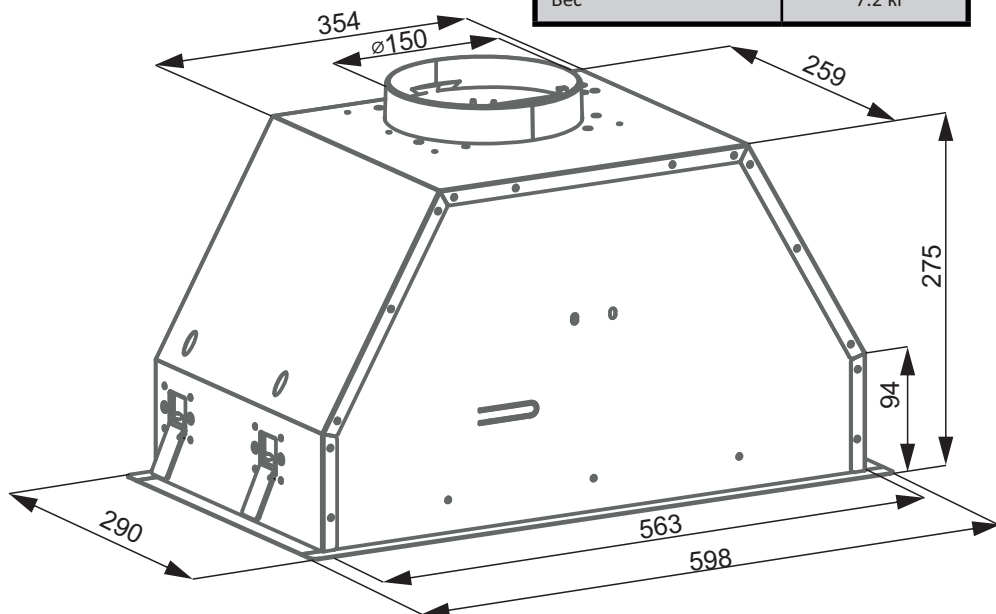
Рис. 1 Внешний вид кухонной вытяжки и схема размеров
